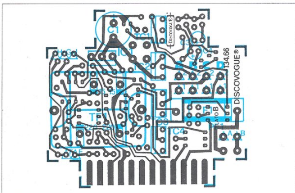
Figura 5. Pista conduttrice del lato B del circuito 134.66 con montaggio dei componenti sul lato B.
